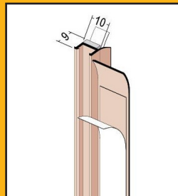
Ikkunalista 9 mm, valkea/musta Monitoiminen tiivisteellä varustettu.
