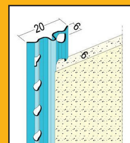
Aloituslista 6 tai 10 mm Rappausohjuri Seinän ja sokkelin rajauksessa käytettävä tippanokallinen lista.
